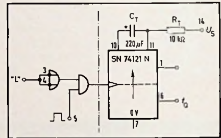
Bild 2. Beschaltung der monostabilen Kippstufe MF 1
