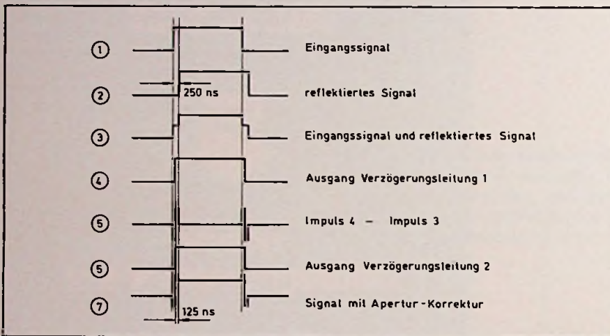
Bild 4. Impulsverhältnisse
