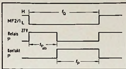
Bild 4. Impulsängen und Entladezeitkonstanten
