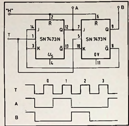
Bild 1. Beschaltung und Impulsdiagramm des Synchronzählers
