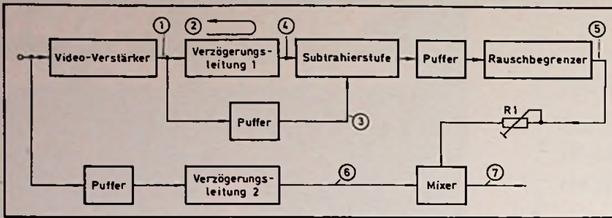
Bild 3. Blockschaltbild Cosinus-Entzerrung
